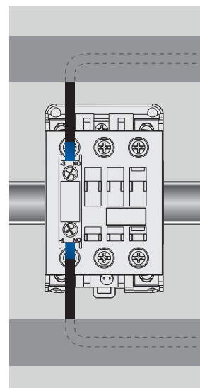
Contatores Padrão
